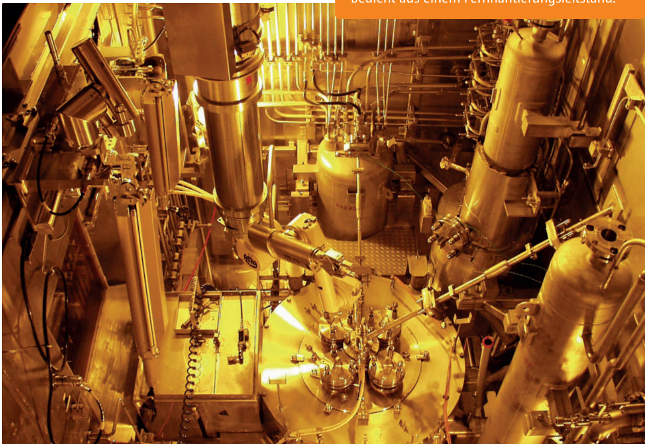
Blick auf den Schmelzofen der Verglasungseinrichtung Karlsruhe (VEK).
