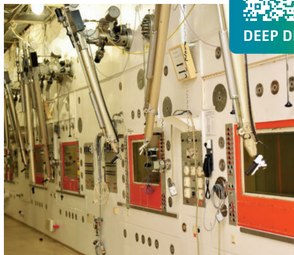
Manueller Rückbau in den Heißen Zellen.
