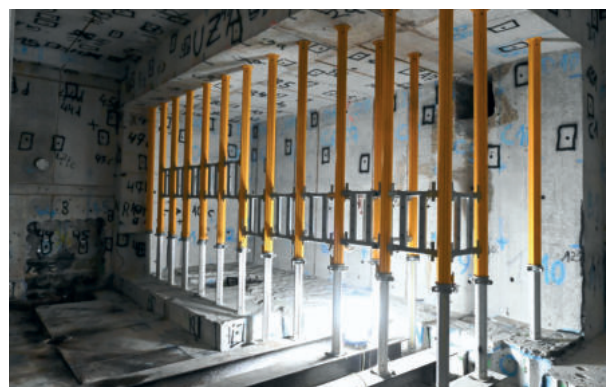
Statische Ersatzmaßnahmen im Hilfsanlagegebäude vor dem Abriss.
